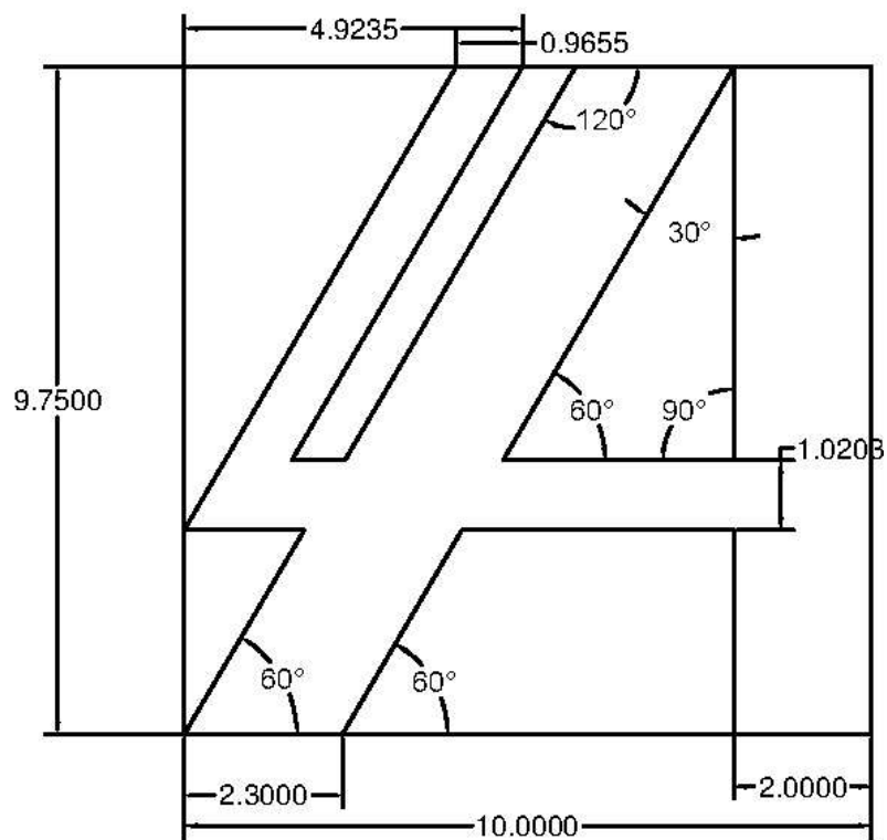
2 pav. Akreditacijos ženklo matmenys
